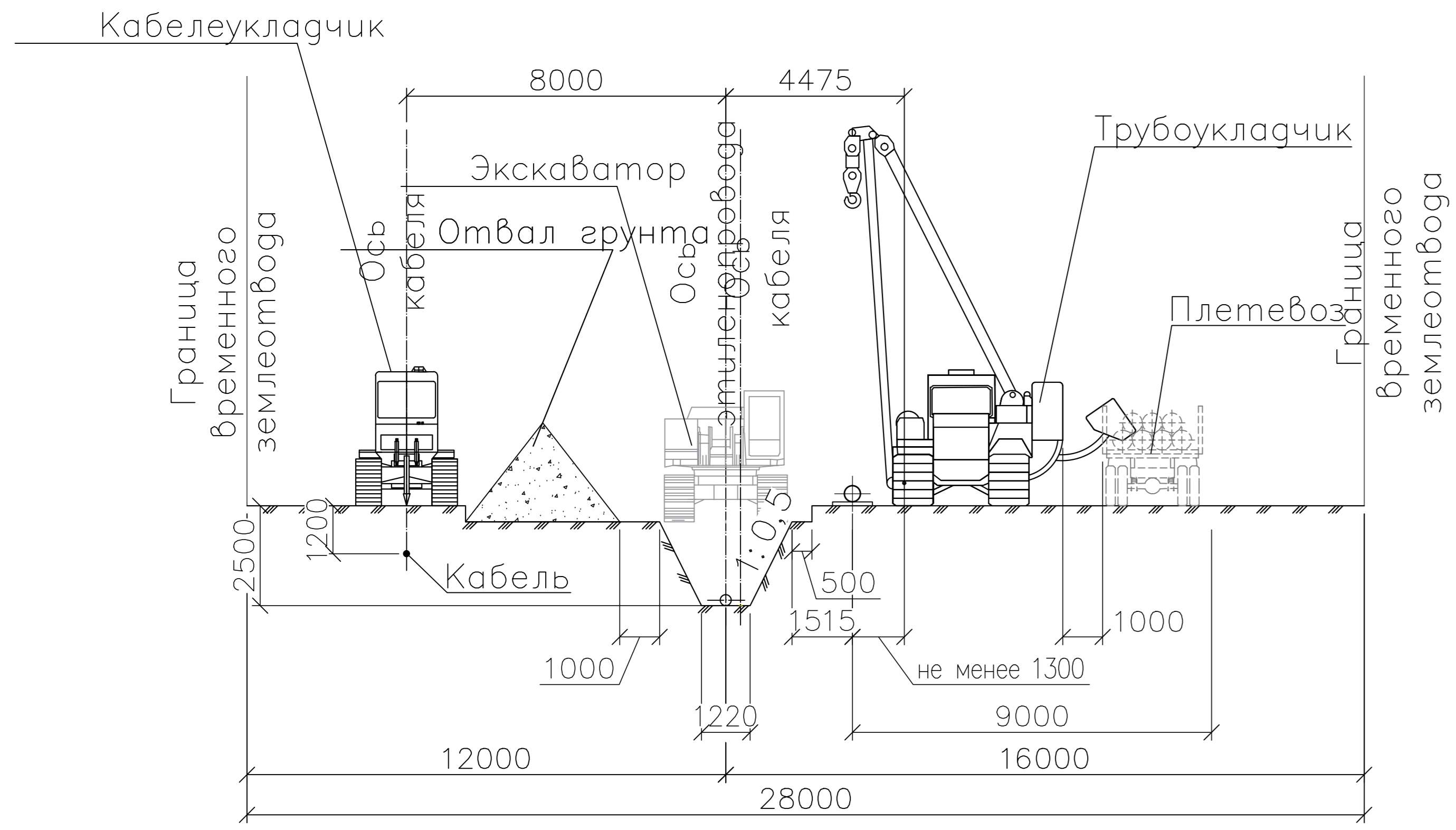
Поперечный профиль полосы отвода при укладке этиленпровода в границах ООПТ и лесопарковых зон
